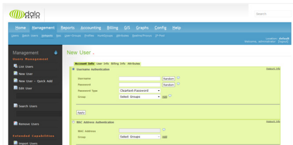
Gambar 14: Tampilan tambah pengguna
